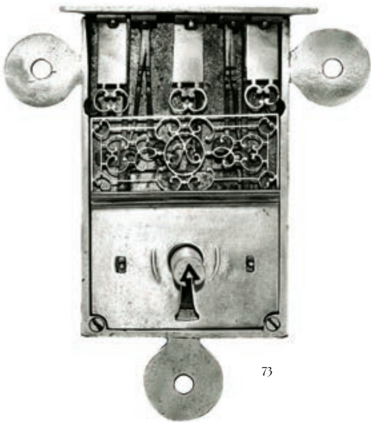
73 Serrure de maîtrise. France, XVIII e siècle. 18 x 11,3 cm - Avec les fixations : 23 x 20 cm
