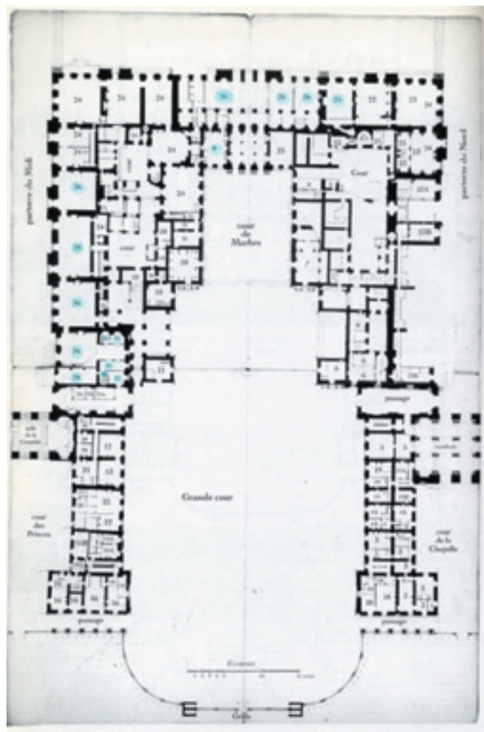
Plan du corps central du château de Versailles au rez-de-chaussée, vers 1752 : en bleu les appartements du Dauphin et de la Dauphine, occupés plus tard par le comte et la comtesse de Provence, Paris, Arch. nat., O 1 1766 1 & n o 1 (d'après W. R. Newton)
